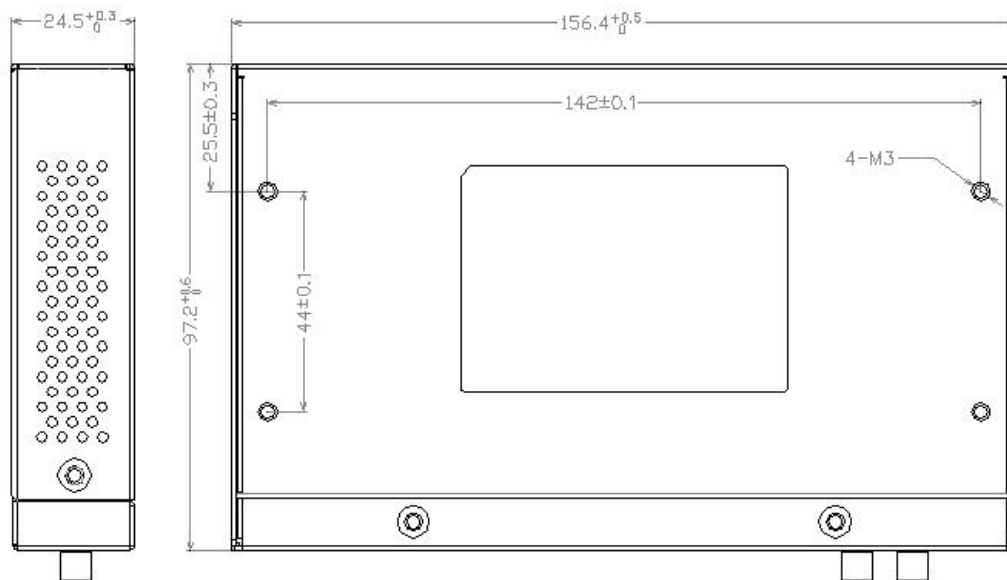
路由器尺寸
