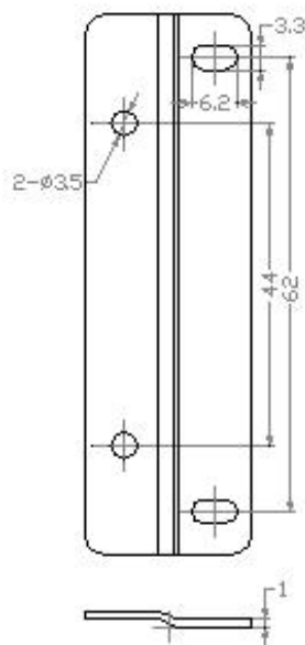
固定片尺寸
